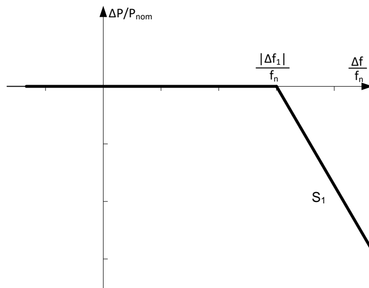
Slika 1 – Sposobnost spremnika energije za frekventijski odziv djelatne snage u slučaju rasta frekvencije
