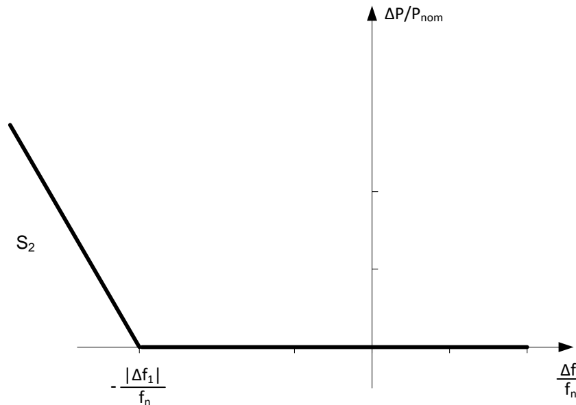
Slika 2 – Sposobnost spremnika energije za frekvencijski odziv djelatne snage u slučaju pada frekvencije
